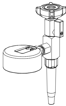
SUCTION - G2040 SCAVENGE - G2050
